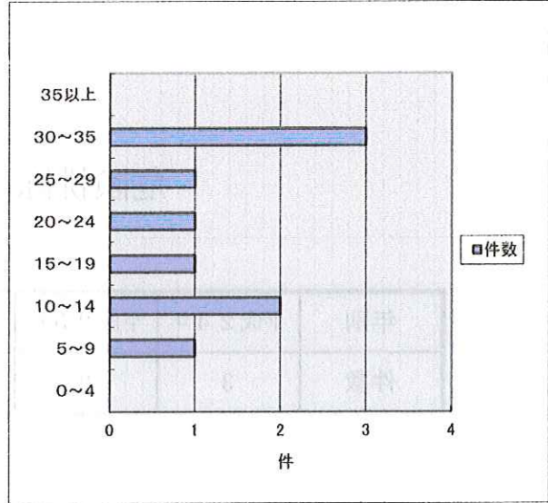
湿度別件数
